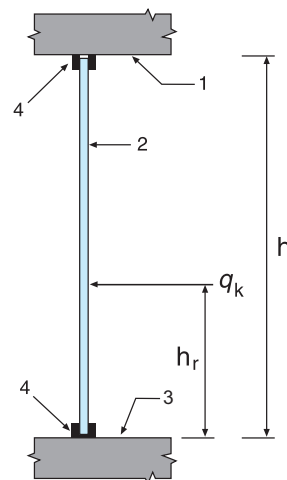
Figur 1 Indvendige fuldglasvægge uden niveauforskel og uden værnfunktion entydigt fastholdt i top og bund
