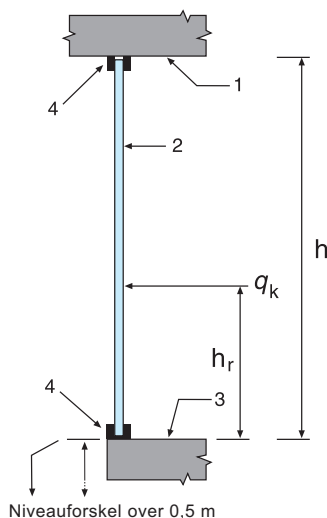
Figur 2 Indvendige fuldglasvægge med niveauforskelle og med værnfunktion entydigt fastholdt i top og bund
